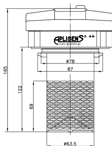
Rysunek gabarytowy SAK-02
