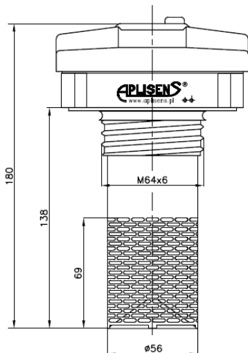
Rysunek gabarytowy SAK-01
